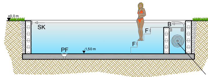
SEZIONE B-B'
