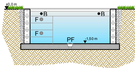
SEZIONE A-A'
