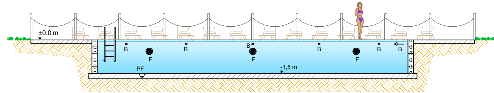
SEZIONE A-A'
