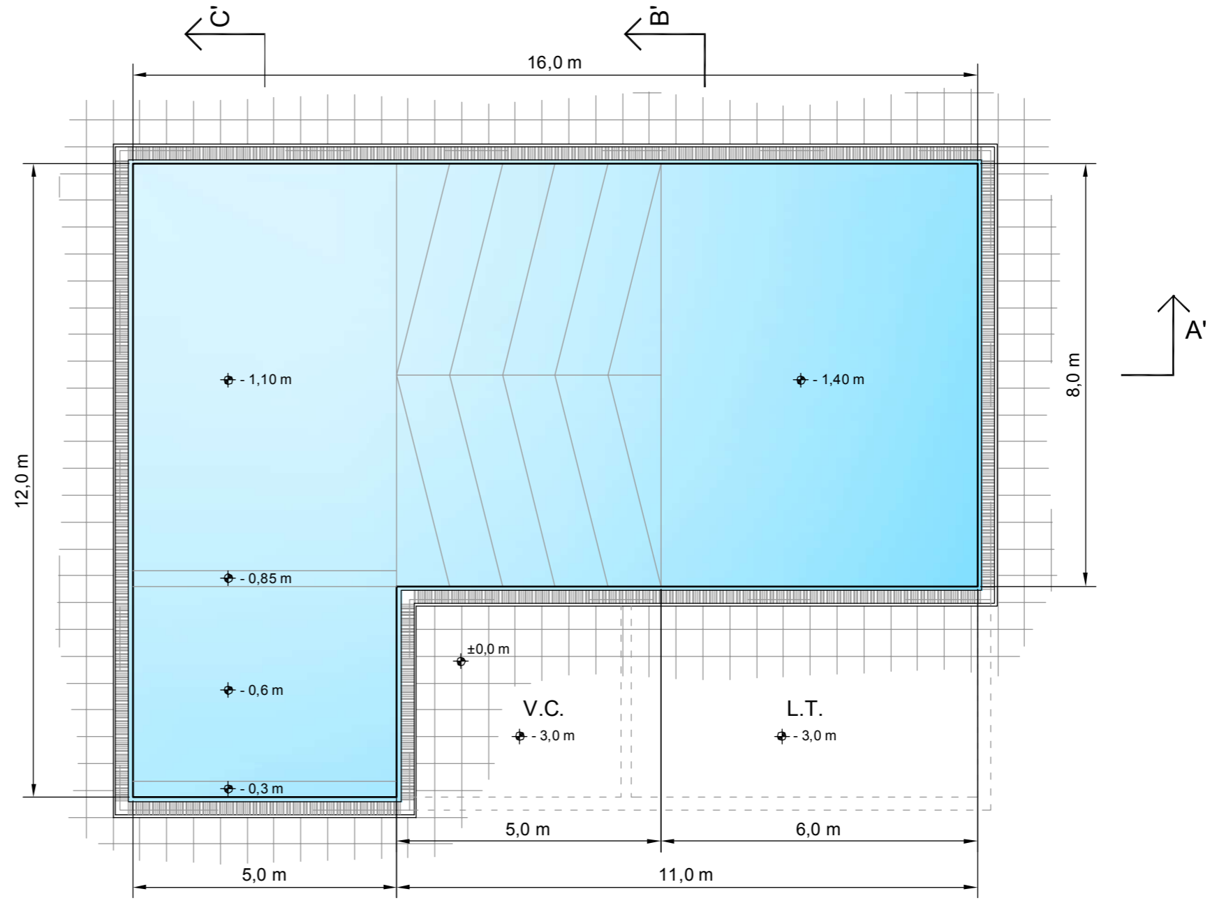
PIANTA
