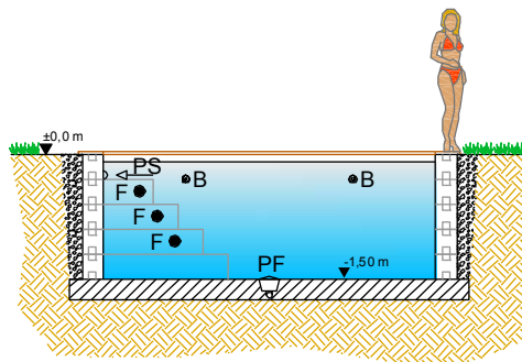
SEZIONE A-A'
