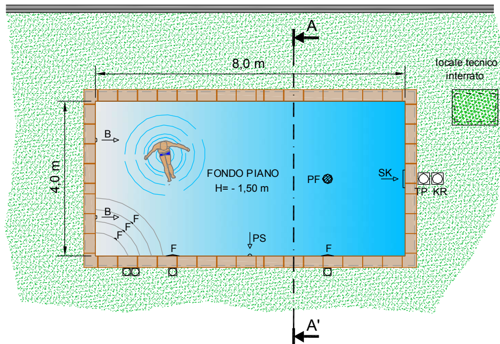
PIANTA
