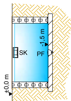
SEZIONE B-B'
