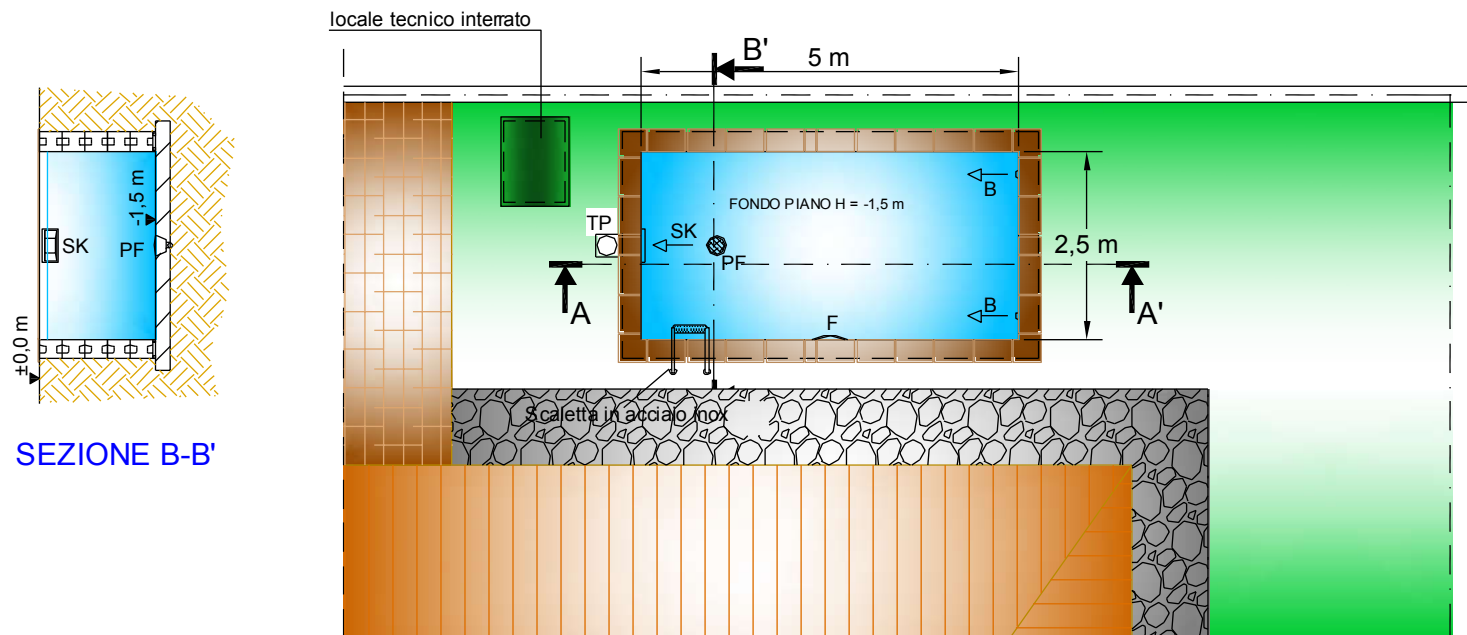
PIANTA
