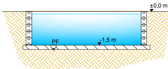
SEZIONE A-A'
