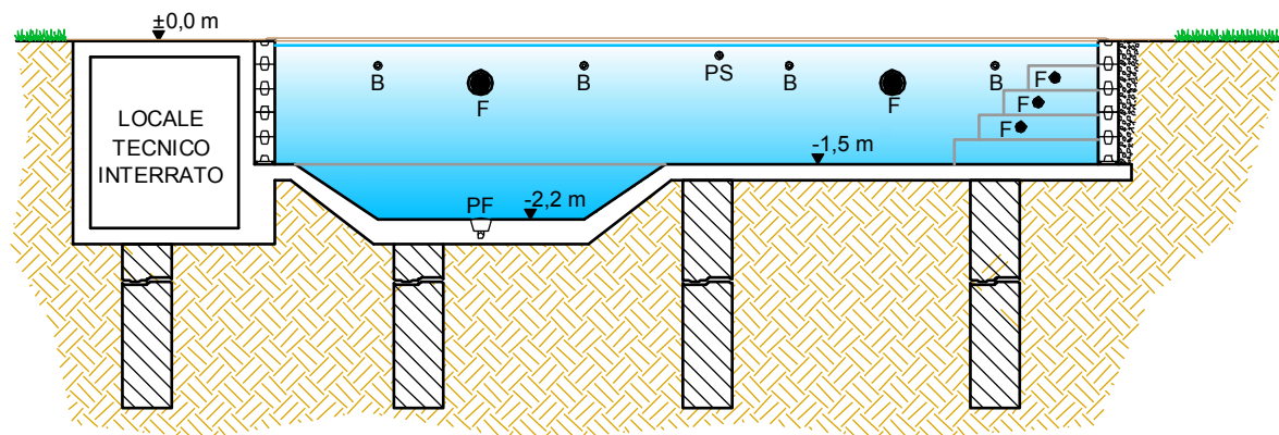
SEZIONE A-A'
