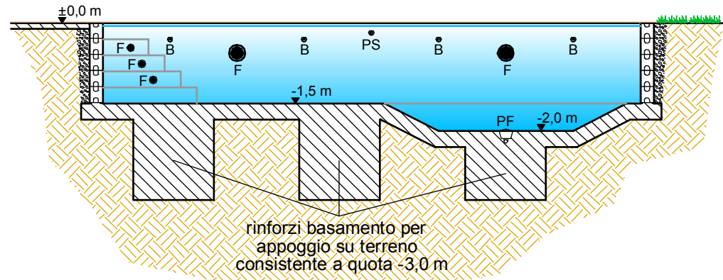
SEZIONE A-A'
