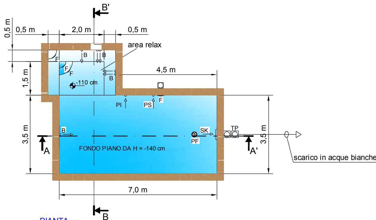
PIANTA
