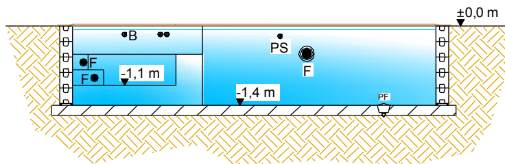
SEZIONE A-A'
