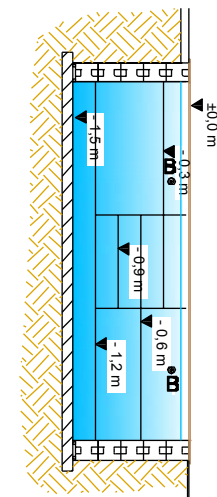
SEZIONE A-A'
