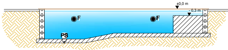
SEZIONE B-B'
