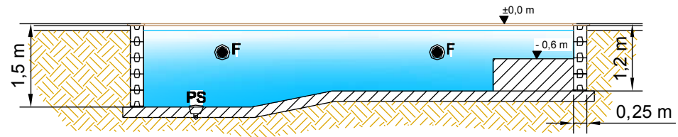
SEZIONE D-D'
