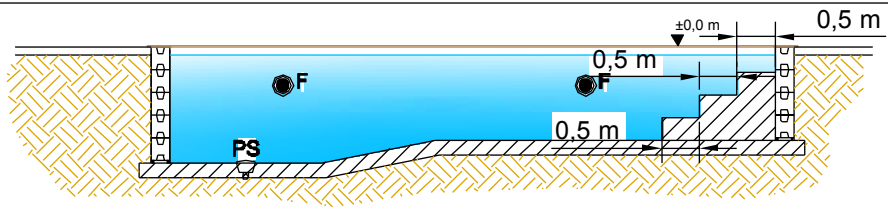
SEZIONE C-C'
